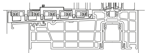
Bodenbündig
