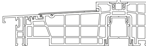
Trittschwelle
