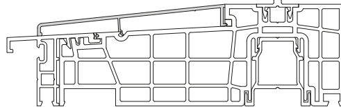
Comfortprofil
